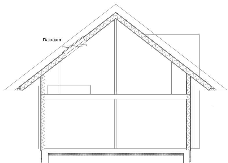
Doorsnede B
