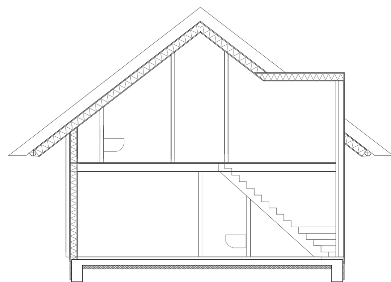
Doorsnede A
