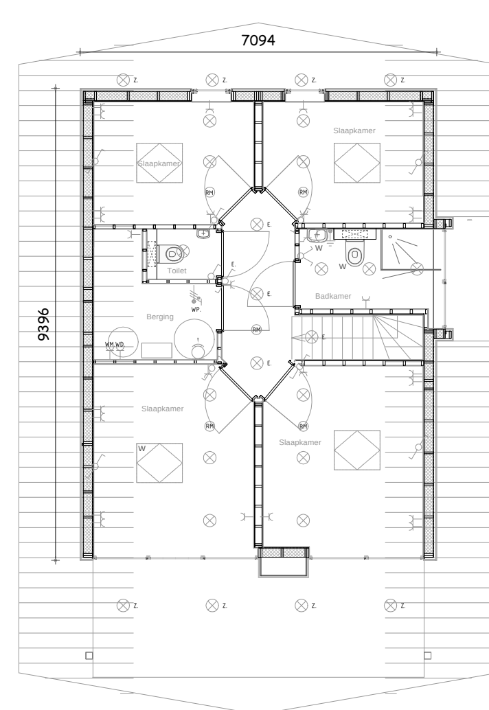
Verdieping
