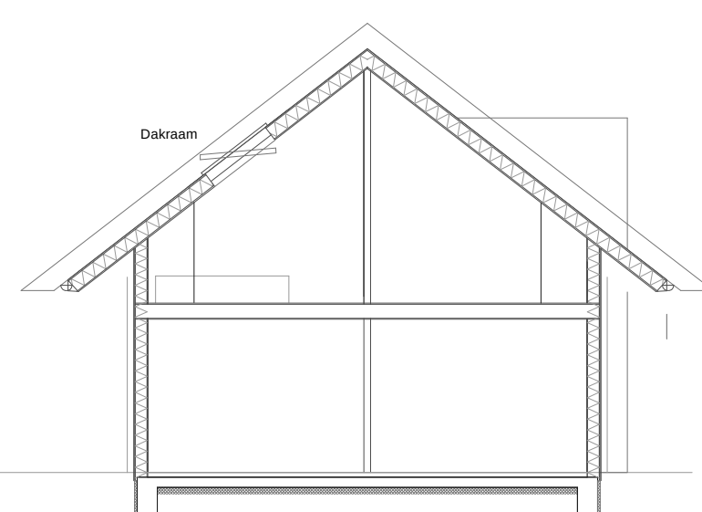
Doorsnede B
