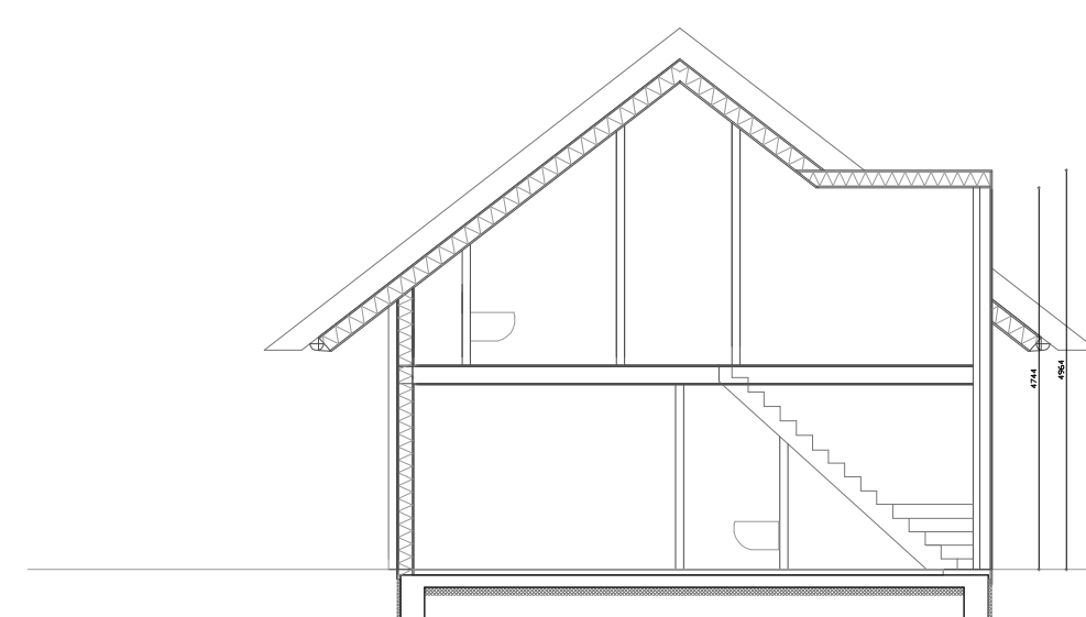
Doorsnede A
