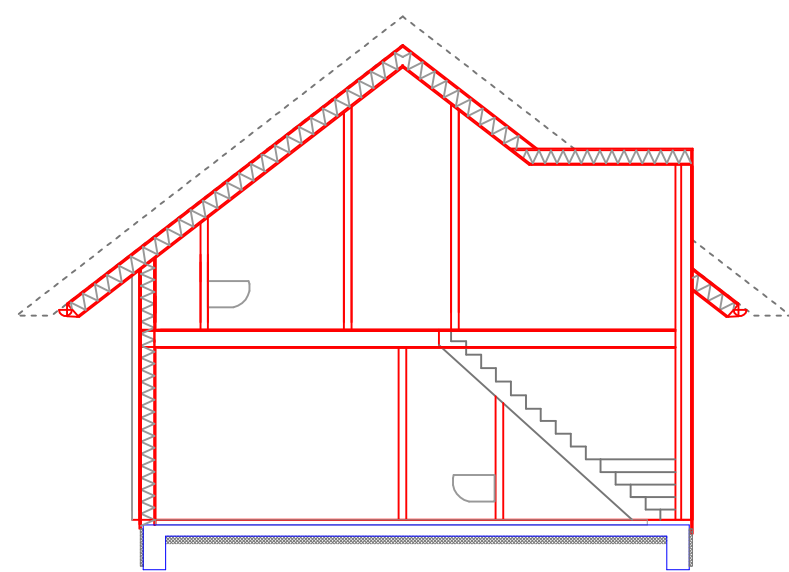
Doorsnede A
