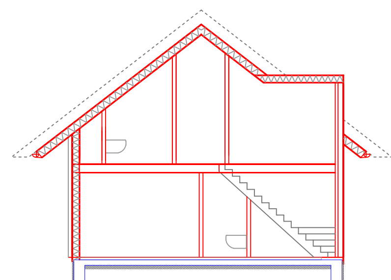
Doorsnede A
