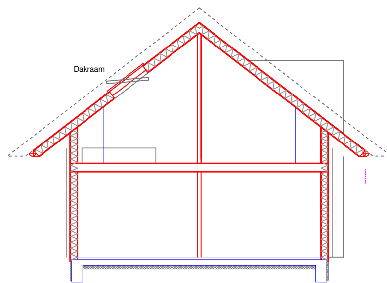
Doorsnede B
