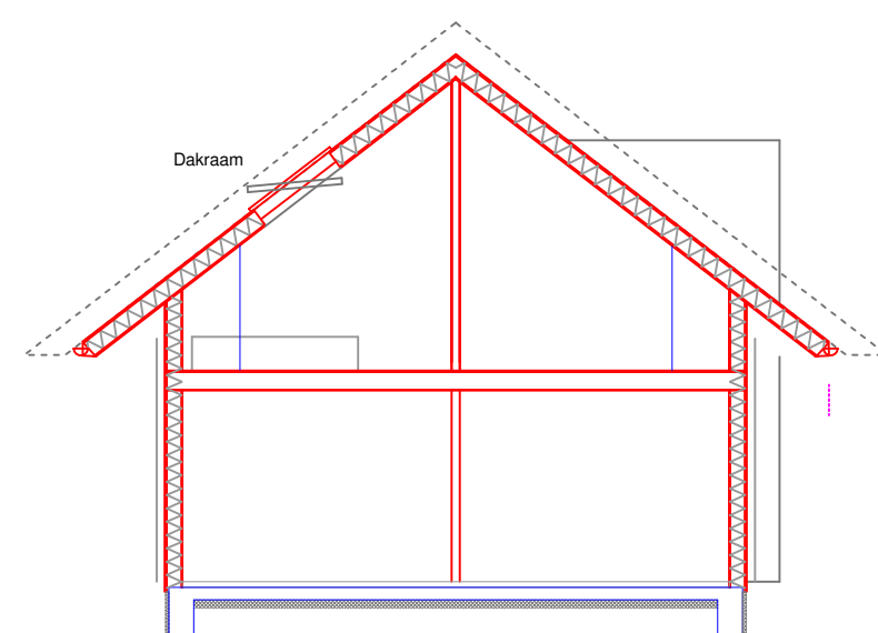
Doorsnede B
